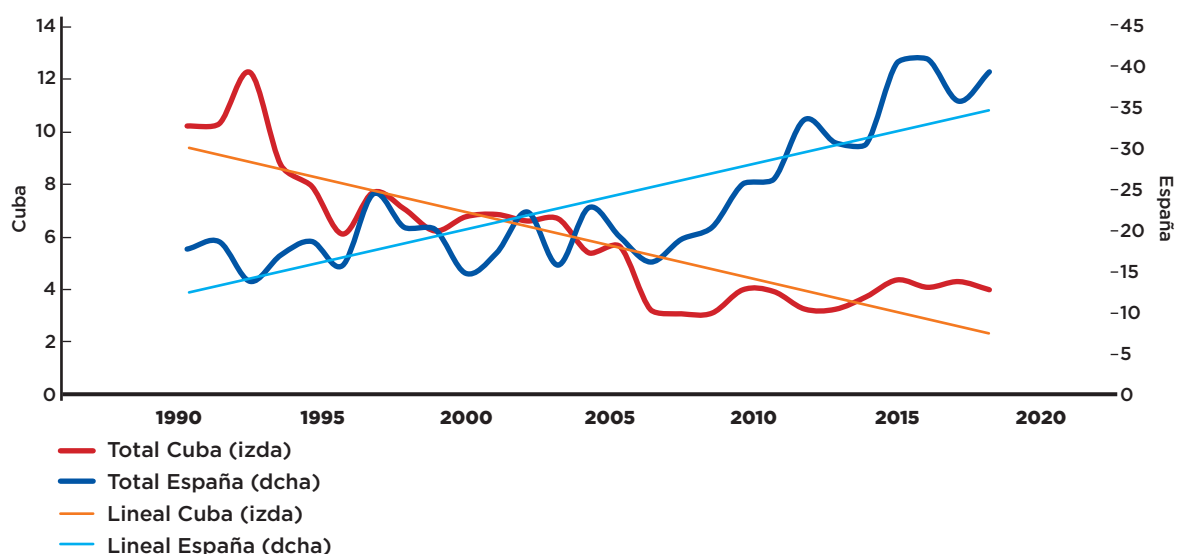
FIGURA 23. PROPORCIÓN DE ELECTRICIDAD PROCEDENTE DE FUENTES RENOVABLES SOBRE TOTAL DE ELECTRICIDAD GENERADA EN CUBA Y ESPAÑA DESDE 1990 HASTA 2016
