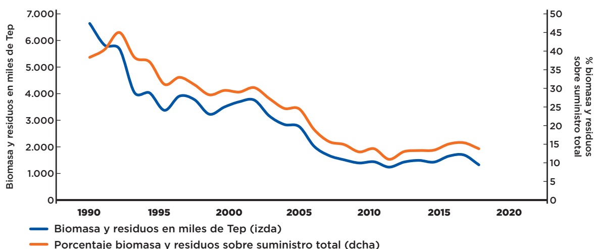
FIGURA 10. BIOMASA Y RESIDUOS Y PORCENTAJE SOBRE CANTIDAD DE ENERGÍA SUMINISTRADA
