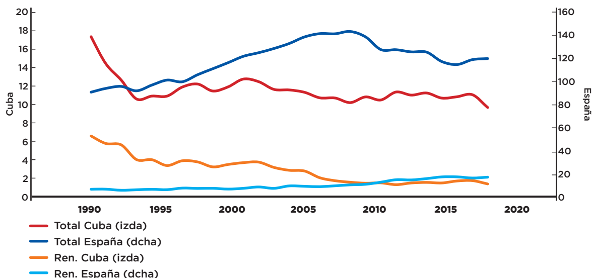
FIGURA 20. SUMINISTRO TOTAL DE ENERGÍA PRIMARIA EN CUBA Y ESPAÑA (EN MTEP) Y SUMINISTRO DE ENERGÍA RENOVABLE (EN MTEP), DESDE 1990 HASTA 2016
