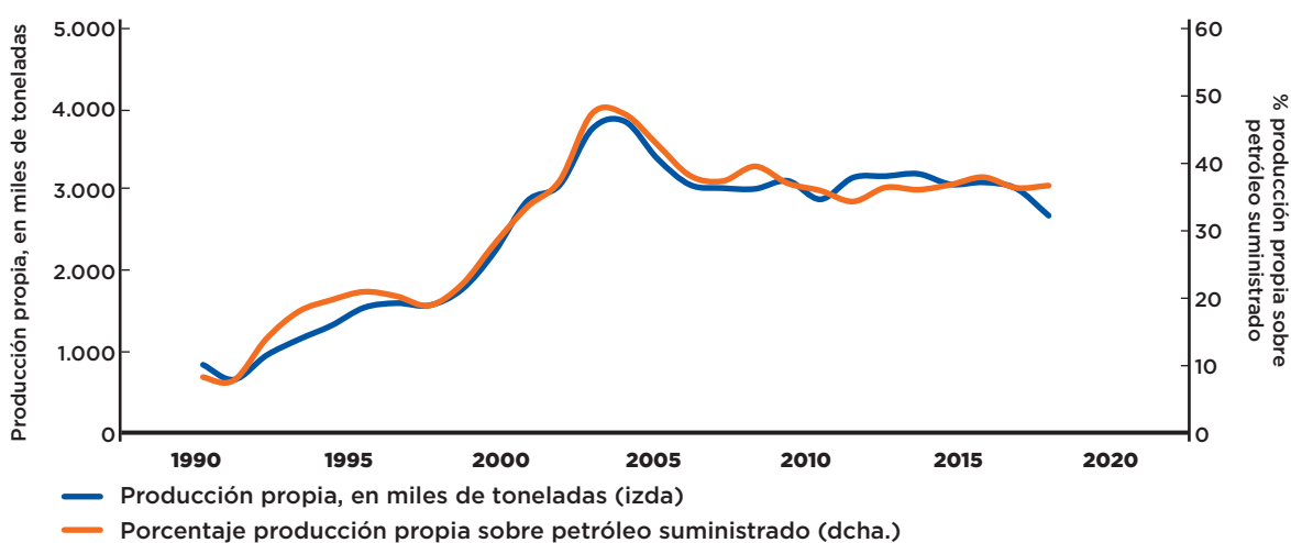
FIGURA 9. PRODUCCIÓN PROPIA DE PETRÓLEO Y PORCENTAJE SOBRE CANTIDAD SUMINISTRADA
