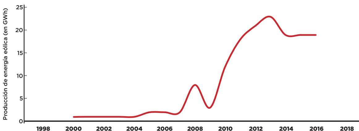
FIGURA 11. PRODUCCIÓN DE ENERGÍA ELÉCTRICA EÓLICA EN CUBA
