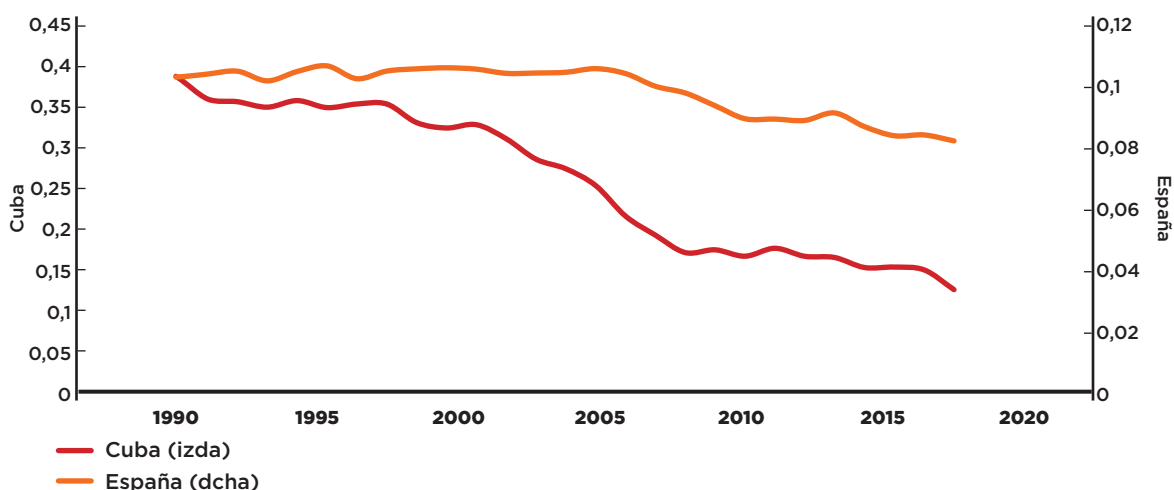
FIGURA 24. INTENSIDAD ENERGÉTICA (TEP/PIB (EN MILES DE 2010 USD) EN CUBA Y ESPAÑA DESDE 1990 HASTA 2016
